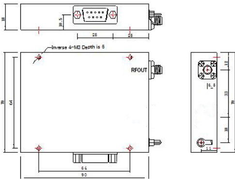
XB-17A UNIT: mm
