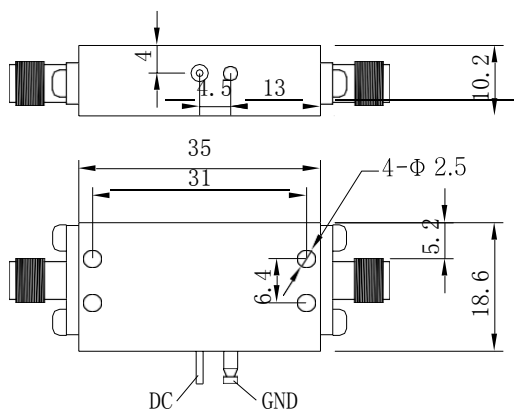
UNIT:mm XB-02A
